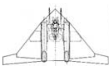
Проект реактивного истребителя Б.И.Черановского
