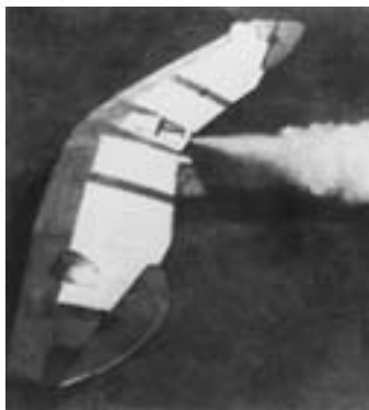
Планер Г.Эспенлауба с ракетным двигателем.
